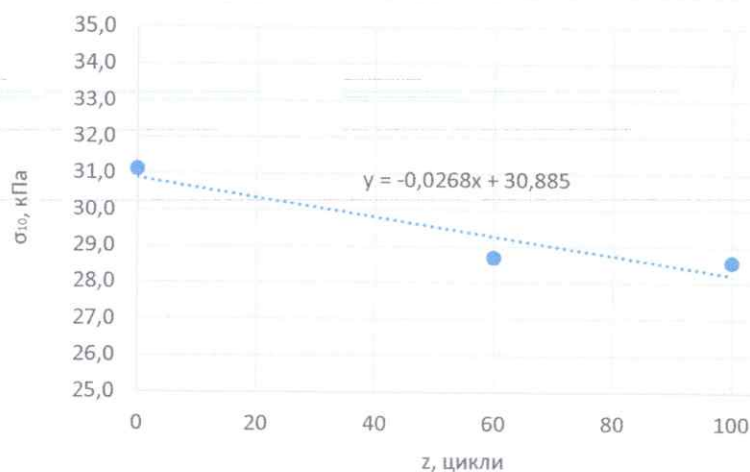
Рисунок 7 – Залежність міцності на стиск при 10% деформації від циклічних впливів зразків № 24/23 теплоізоляційного матеріалу марки «ТЕХНОРУФ Н ЕКСТРА»
